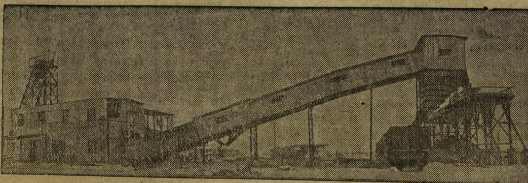
Общий вид шахты № 1 треста „Домбаровуголь“.
